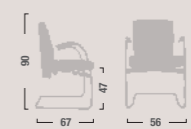
TK36 Sedia fissa con braccioni. Fixed armchair.
